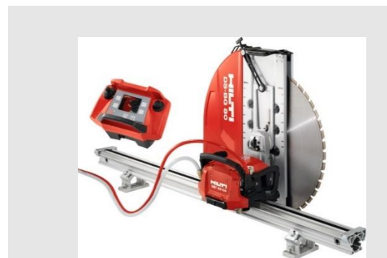
遙控牆鋸
