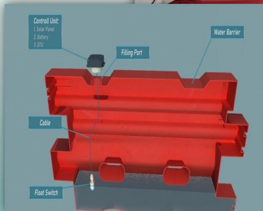
水位監察器 (即時監測水馬水位)
